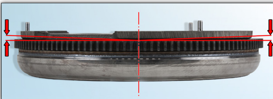
Bild 2: Das Kippspiel der Sekundärmasse stellt keinen Mangel dar
