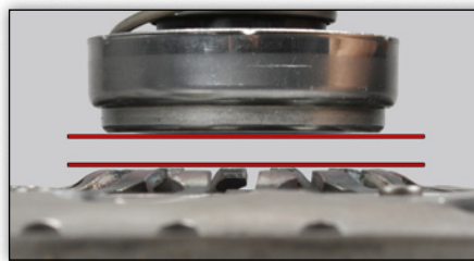
Bild 3: korrekter Einbau
